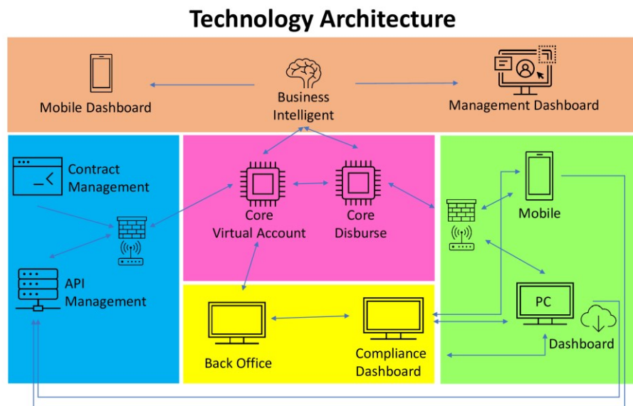
Gambar 5. Arsitektur Teknologi
