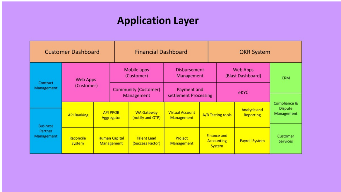
Gambar 3. Arsitektur aplikasi terhadap industri fintech
