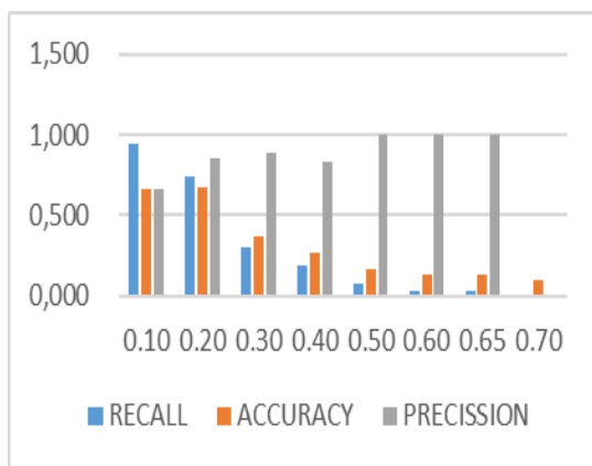
Gambar 6. Grafik perhitungan precision , recall , dan accuracy
