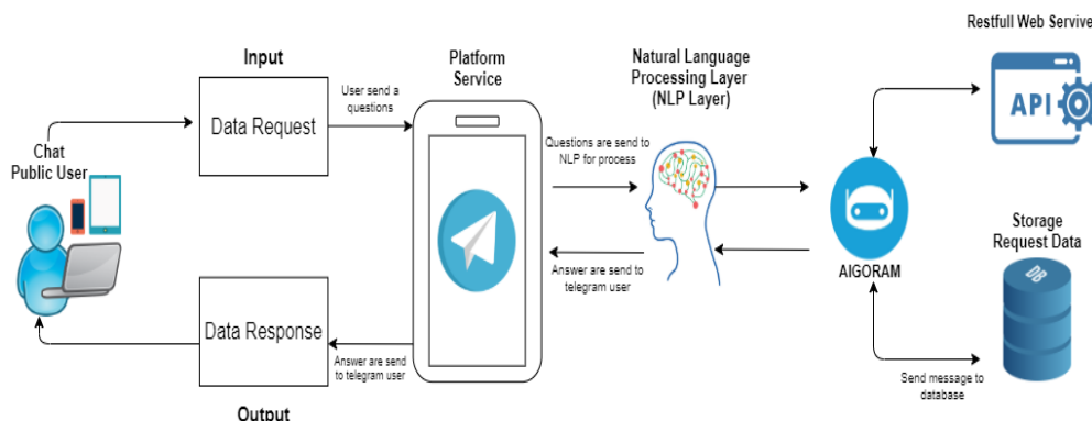
Gambar 2. Ilustrasi sistem bot
