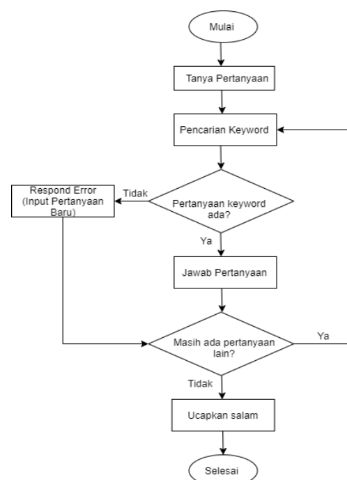
Gambar 1. Flowchart chatbot aplikasi
