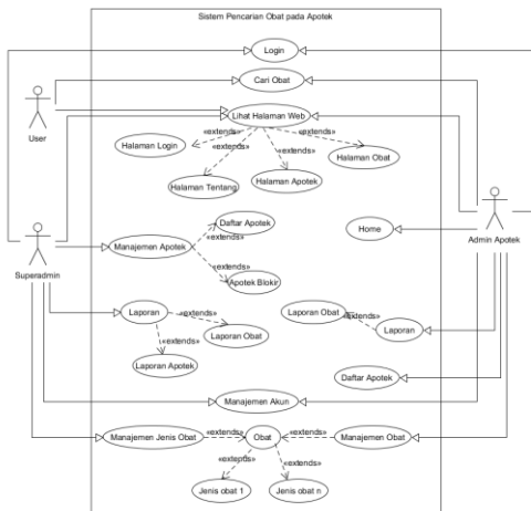
Gambar 2 : Use Case Diagram Sistem Pencarian Obat pada Apotek
