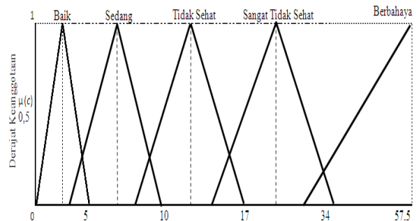
Gambar 4. Derajat keanggotaan variabel SO 2
