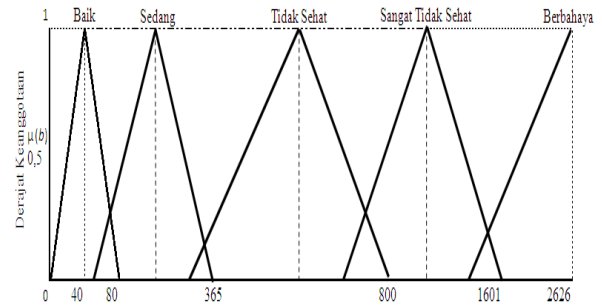
Gambar 4. Derajat keanggotaan variabel SO 2
